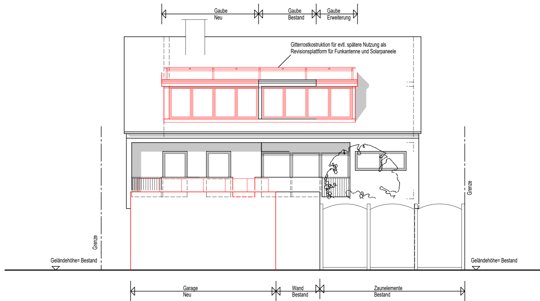
Ansicht Süd
